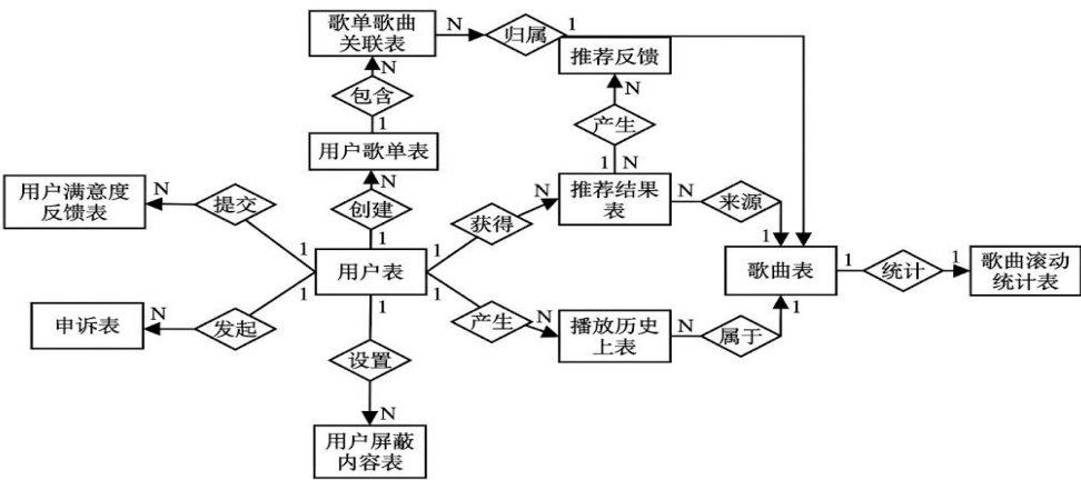
图 4-4 系统核心实体关系图
